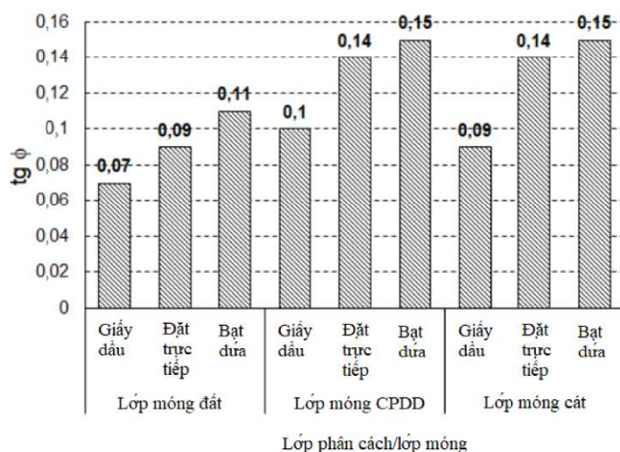
Hình 5. Ảnh hưởng của vật liệu lớp phân cách và lớp móng tới tan \phi
